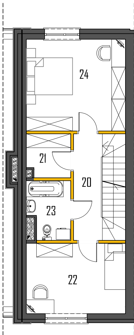
RZUT PODDASZA
